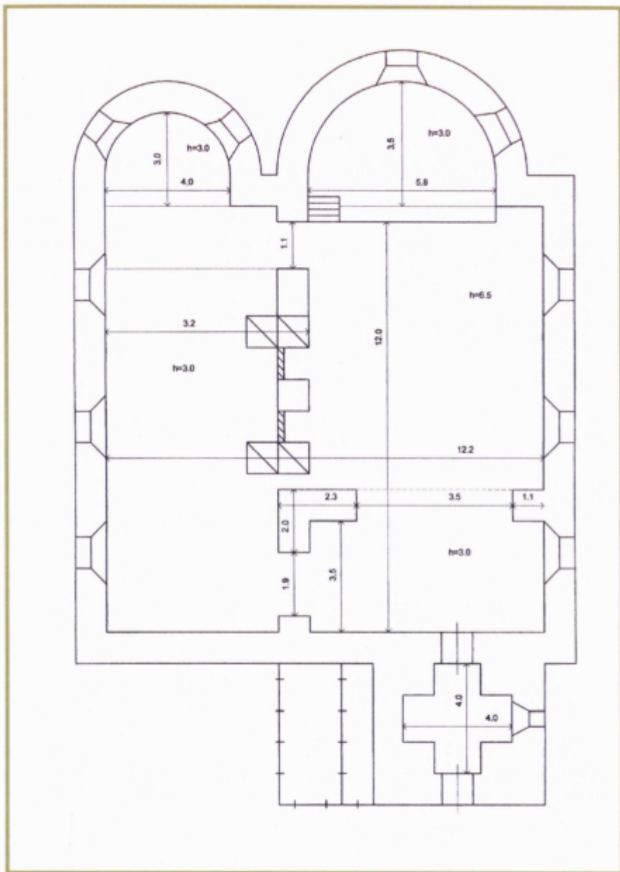
План - чертёж летней церкви с колокольней.
